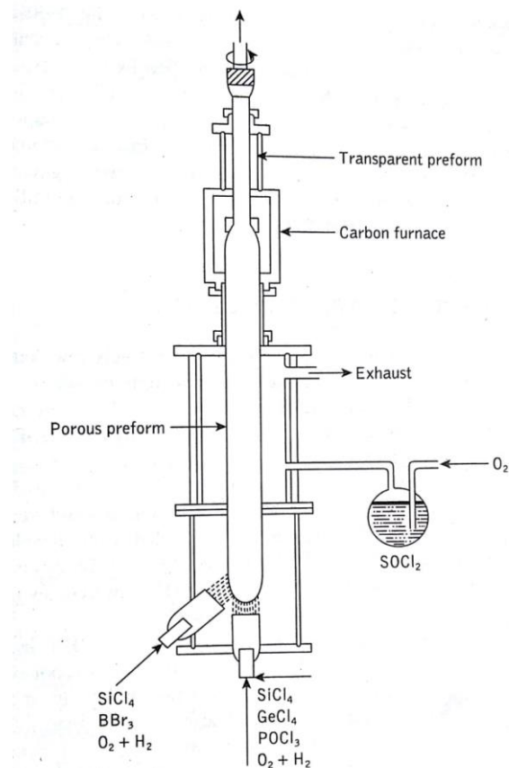
Fig: VAD Process
